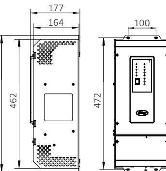
Zijaanzicht
