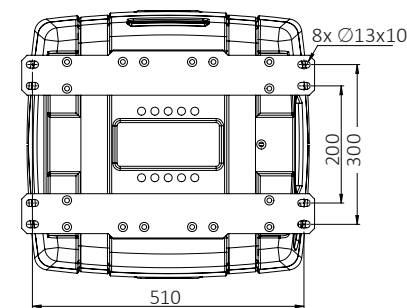
Onderzijde
