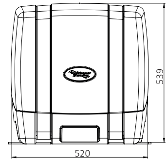
Vooraanzicht
